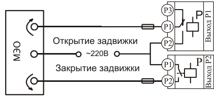
Подключение электродвигавки
